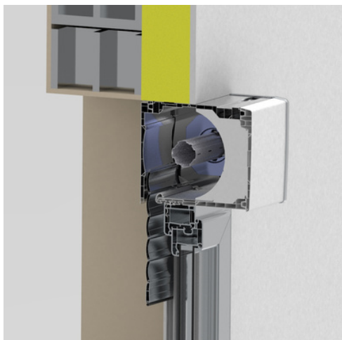
Volet roulant bloc baie
