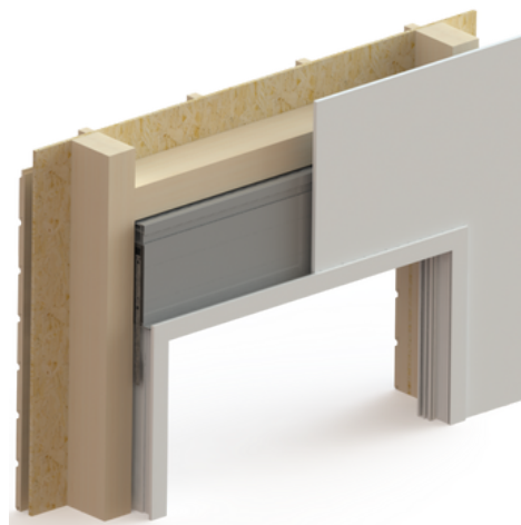
Volet roulant demi-linteau
